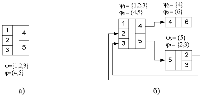
Рис. 3. Пример отдельного узла (а), а также сети из нескольких связанных узлов (б). Идентификаторы в левой части изображения узла соответствуют входным сигналам, а в правой части – выходным. Связи между узлами показаны стрелками
