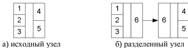
Рис. 5. Пример работы оператора разделения узла
