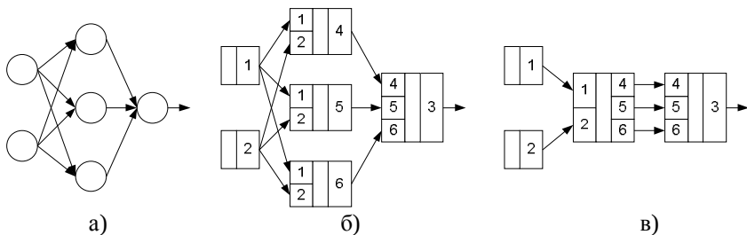
Рис. 4. Пример использования РС для компактной записи информации о структуре ИНС: а) структура ИНС; б) соответствующая РС; в) РС с объединенными по входам узлами
